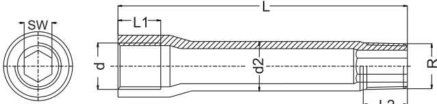
Steel Extension Tube / Verlängerungsrohr aus Stahl
