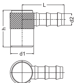
Flexible Diverting connector / Umlenkupplung mit Schnellsteck- Schlauchtülle
