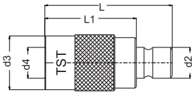
Adapting Socket with Plug Adapterkupplung mit Nippel
