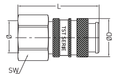
Female Thread Coupling Kupplung mit Innengewinde
