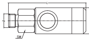
Male Thread Coupling Kupplung mit Aussengewinde
