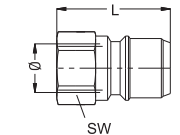
Plug With Female Thread Nippel mit Innengewinde
