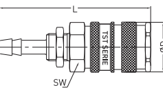
Panel Mount Standard Plastic Hose Coupling Kupplungen mit Schottverschraubung Schlauchanschluss
