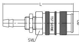
Panel Mount Plastic Hose Coupling Kupplung mit Schottverschraubung Schlauchanschluss
