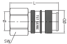
Female Thread Coupling Kupplung mit Innengewinde
