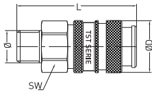
Male Thread Coupling Kupplung mit Aussengewinde
