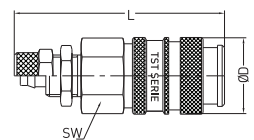
Panel Mount Plastic Hose Coupling Kupplung mit Schottverschraubung für Kunststoffschlauch
