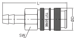
Standard Hose Barb Coupling Kupplung mit Schlauchtülle
