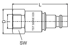
Female Thread Shut-off Plugs Nippel mit Innengewinde
