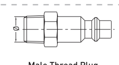
Male Thread Plug Nippel mit Aussengewinde
