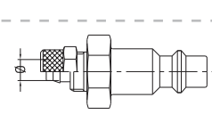
Plastic Hose Plug Nippel für Kunststoffschlauch
