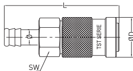
Standard Hose Barb Coupling Kupplung mit Schlauchtülle
