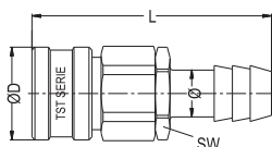
Standard Hose Barb Socket Kupplung mit Schlauchtülle
