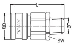
Conical Male Thread Socket Kupplung mit Aussengewinde
